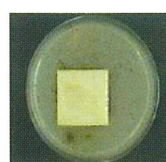
MVX塗布板 カビ菌添加4週間後
